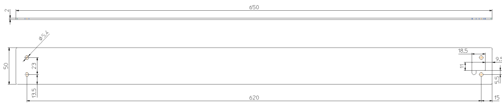
Abmessungen PK00578 (VBlech 600) Material Edelstahl
